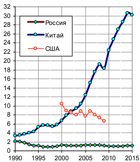
Рис. 1.144, г. Производство каустической соды (100%), млн. т. Источники: [1.3, 1.6]; National Bureau of Statistics of China; Statistics Bureau, The 2012 Statistical Abstract.
