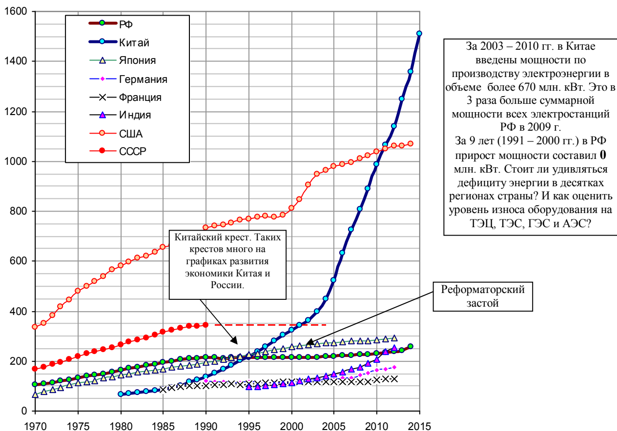
Рис. 1.124, а. Установленная мощность электростанций, млн. кВт. Источники: [1.4, 1.6]; National Bureau of Statistics of China; Japan Statistical Yearbook; U.S. Energy Information Administration (EIA), International Energy; U.S. Census Bureau, Statistical Abstract.
