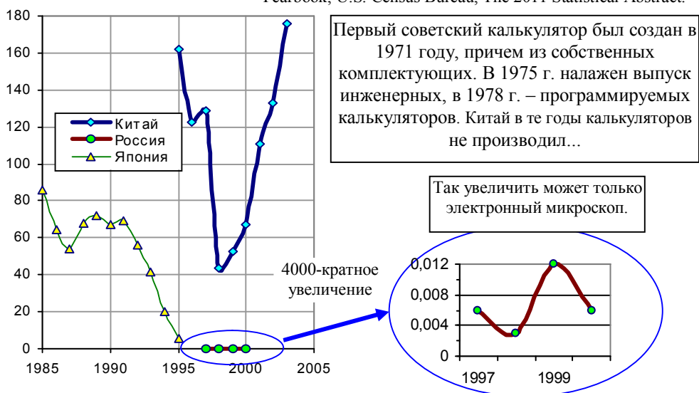
Рис. 1.201. Производство персональных компьютеров в России и в Японии, микрокомпьютеров (micro-computers) и ноутбуков в Китае, отгрузка ПК в США, млн. шт. Источники: [1.6]; National Bureau of Statistics of China; Japan Statistical Yearbook; U.S. Census Bureau, The 2011 Statistical Abstract.
