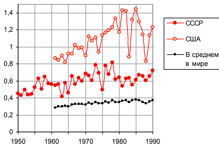
Рис. 1.340, а. Производство зерновых на душу населения в некоторых странах мира, тонн/чел. Источники: [I.6, I.31 – I.33]; расчет по данным FAO.
