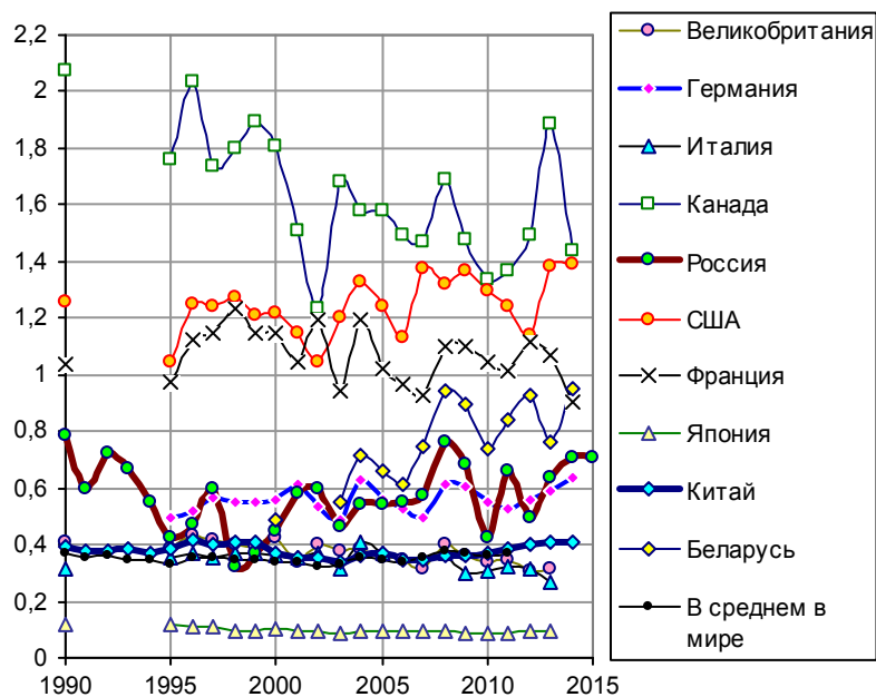
Рис. 1.340, б. Производство зерновых (cereals) на душу населения в некоторых странах, тонн/чел. Источники: [I.6, I.31 - I.33]; National Bureau of Statistics of China; FAOSTAT.
