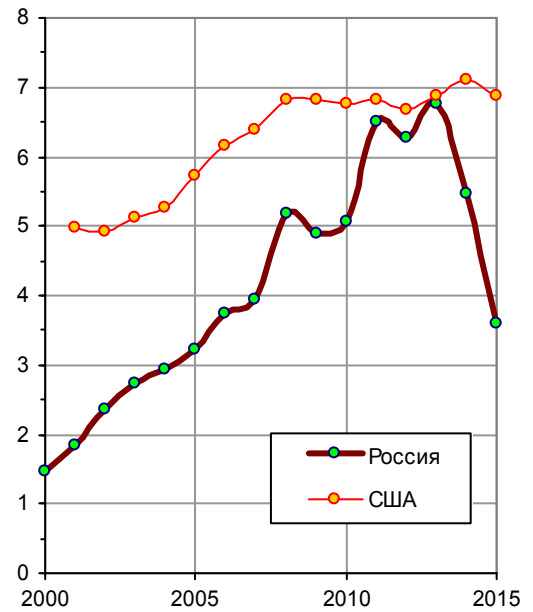
Рис. 1.128, б. Средняя цена в центах за 1 кВт·ч на приобретаемую промышленными предприятиями электроэнергию. Источники: Росстат [1.6]; U.S. Energy Information Administration, EIA. Для России данные на конец года в рублях пересчитаны в центы США по среднегодовым курсам.
